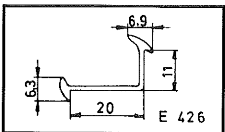
⑧ Winkelprofil für Kantenleiste E 426
