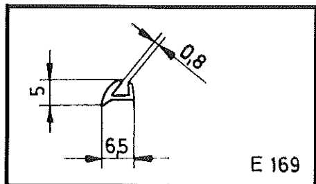
⑥ Unterlegprofil (Leistenschuh) E 169 für Friesleiste u. Abdeckleiste
